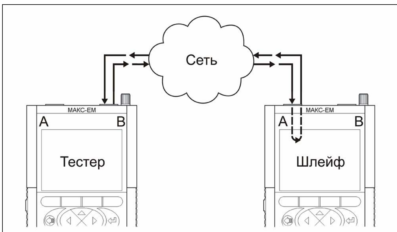
Рис. 9.1 Схема подключения приборов в режиме тестирования
